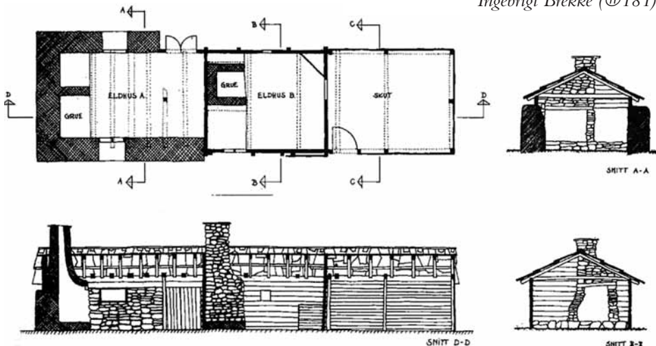
182 Eldhusa på Nerheim. Plan og snitt.
