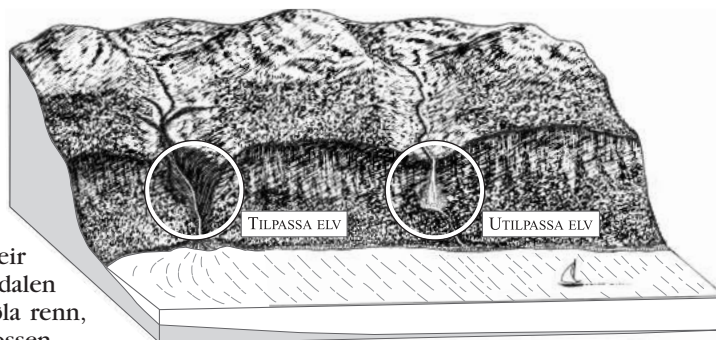
Skilnaden mellom ei tilpassa og ei utilpassa elv. (Wojtek Nemeć)
